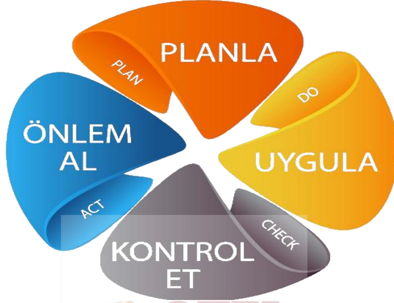
Şekil 1. PUKÖ Döngüsü
